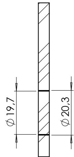
PRZEKRÓJ C-C
